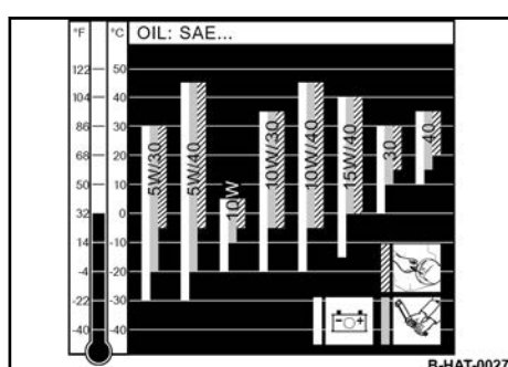
Bild 50: Oljeviskositetsdiagram
